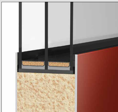
3-fach-Wärmeschutzglas
